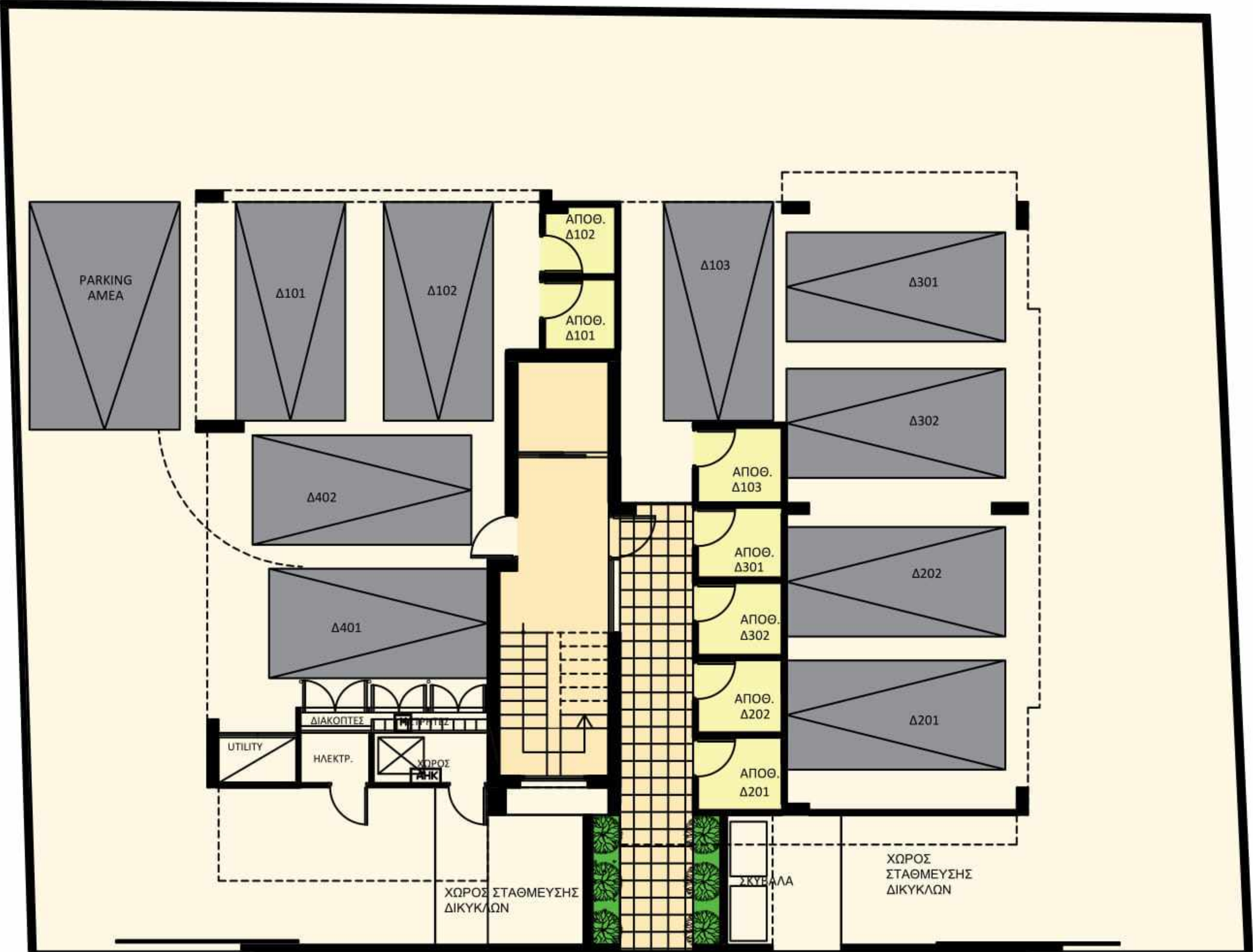
ΚΑΤΟΨΗ ΥΠΟΣΤΕΓΟΥ
